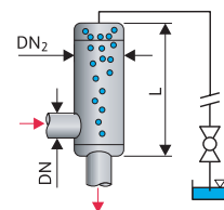
Вертикальный монтаж
