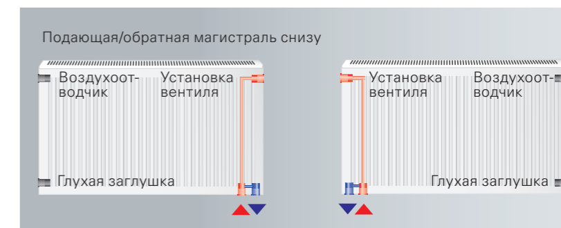
Вентильные радиаторы отопления, вариант подключения как вентильных радиаторов
