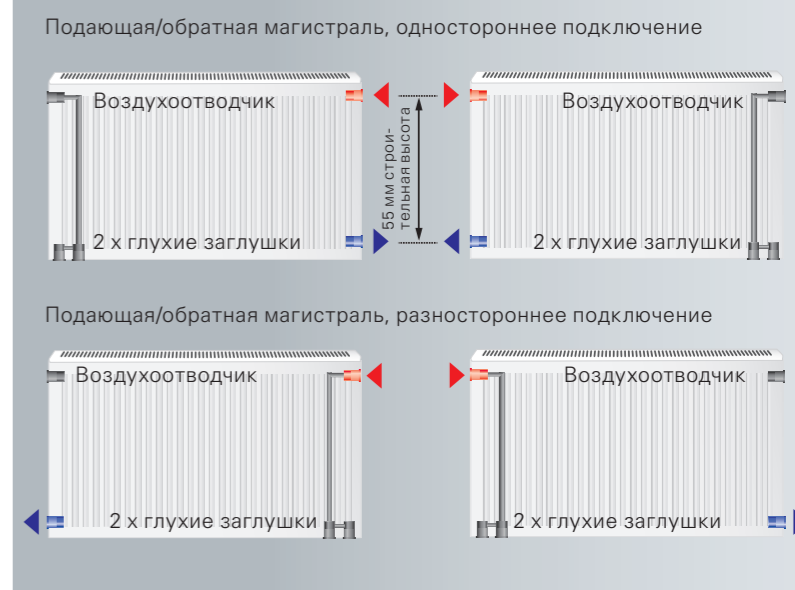
Компактные радиаторы отопления, варианты подключения как для компактных радиаторов
