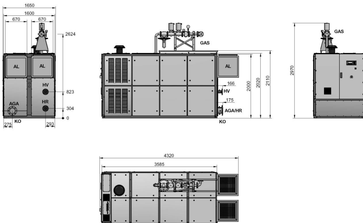
Рис. 1 Размеры и подключения модулей БТЭС Vitobloc 200 EM-238/363 (размеры в мм); уже смонтированный вентиляторный блок на обратной стороне можно демонтировать для установки модуля
