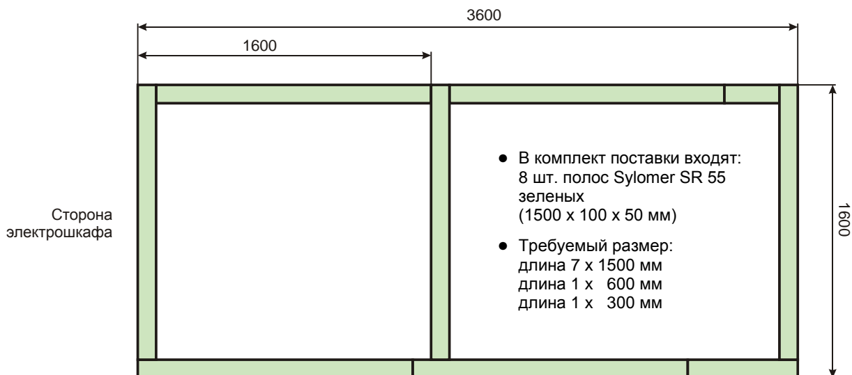
Рис. 5 План укладки полос Sylomer
