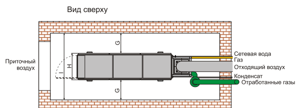
Рис. 9 Подача приточного воздуха в рабочее помещение и отвод отходящего воздуха
