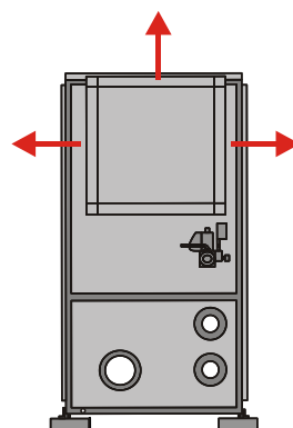
Рис. 10 Возможности подключения для выпускного канала
