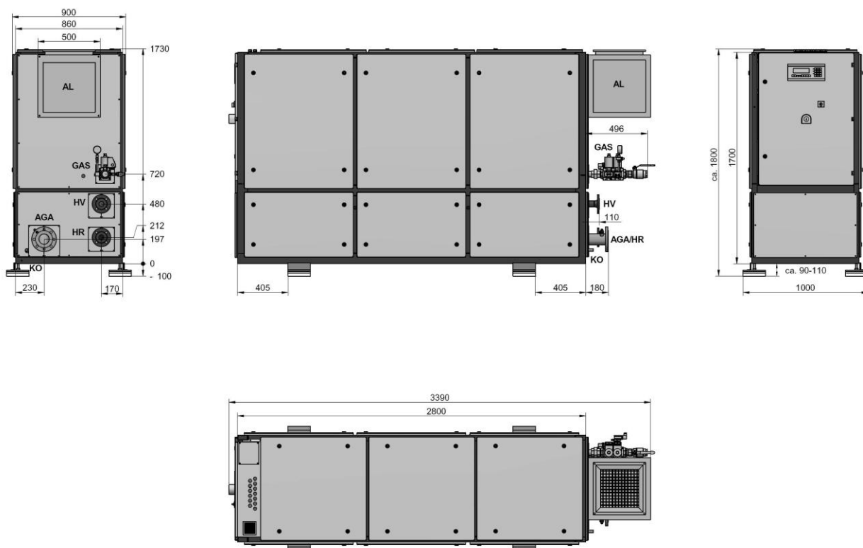
Рис. 1 Размеры и подключения модулей БТЭС Vitobloc 200 EM-70/115 (размеры в мм); уже смонтированный вентиляторный блок на обратной стороне можно демонтировать для установки модуля
