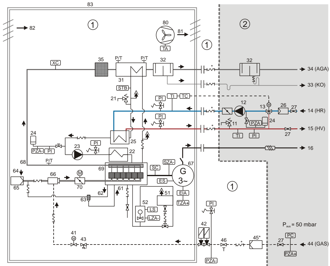
Рис. 8 Технологическая схема модуля БТЭС с возможностями периферийного подключения
