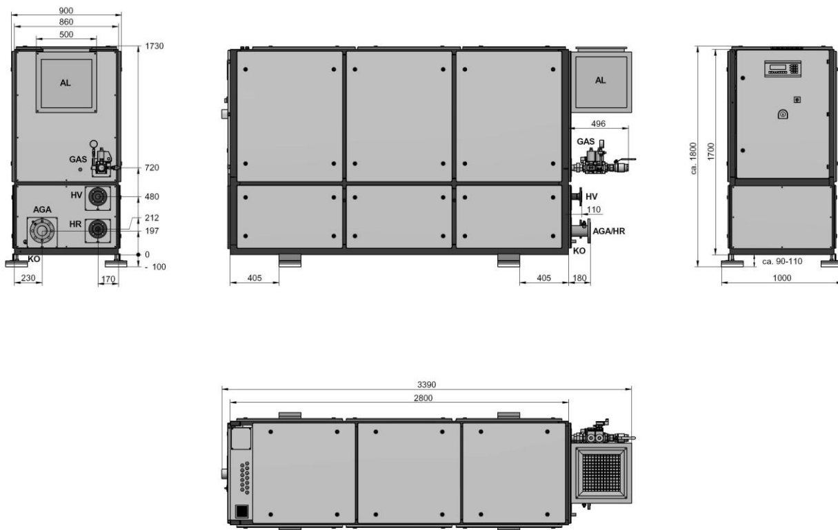
Рис. 1 Размеры и подключения модулей БТЭС Vitobloc 200 EM-50/81 (размеры в мм); уже смонтированный вентиляционный блок на обратной стороне можно демонтировать для установки модуля.
