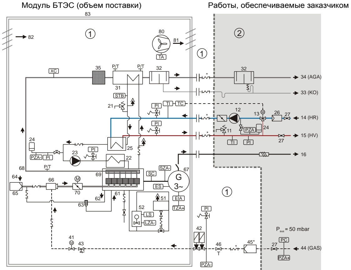
Рис. 2 Контрольные устройства
