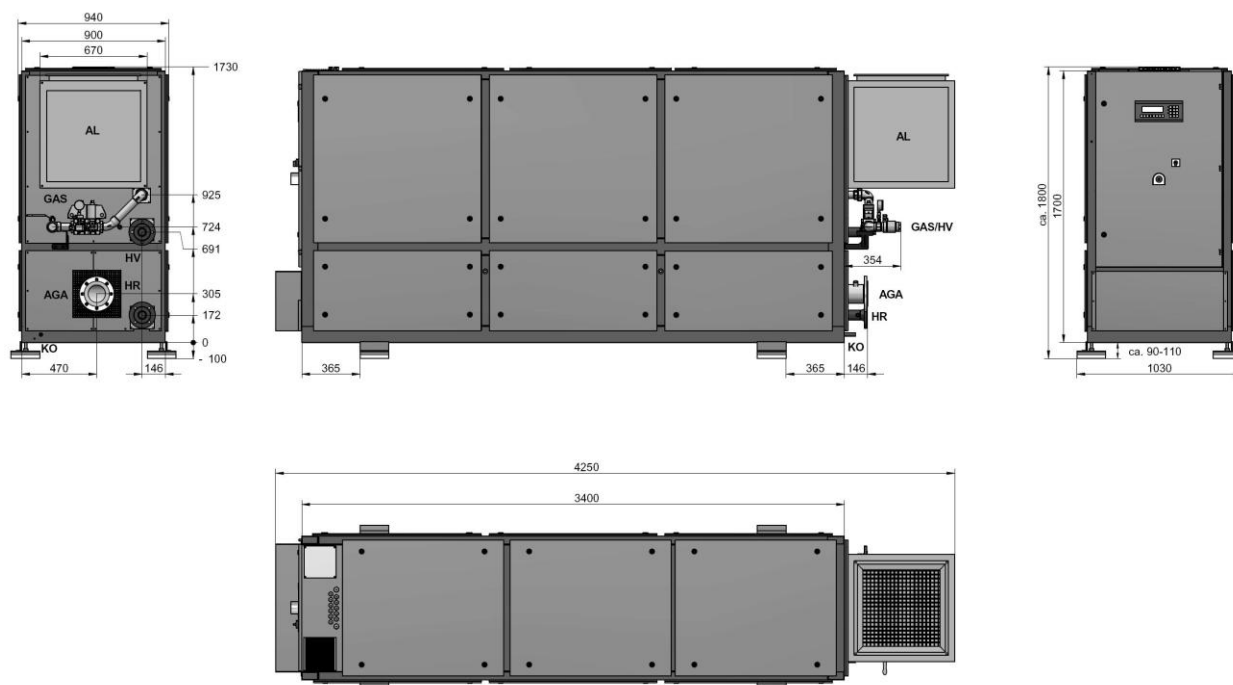
Рис. 5 Размеры и подключения модулей БТЭС Vitobloc 200 EM-140/207 (размеры в мм); уже смонтированный вентиляторный блок можно демонтировать для установки модуля
