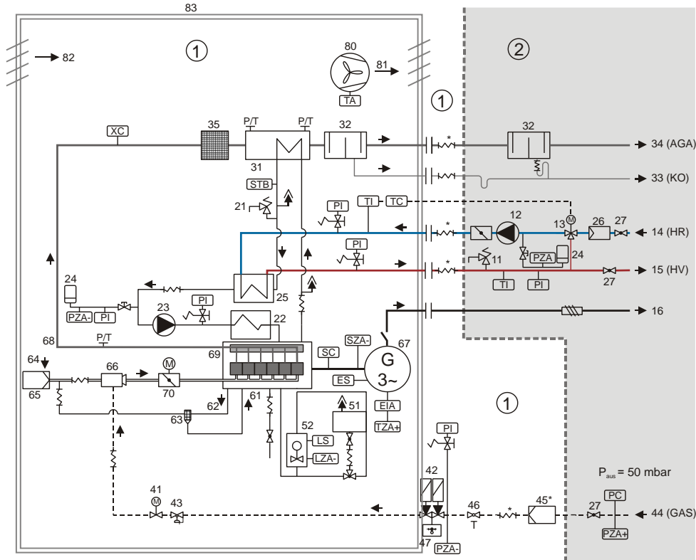
Рис. 2 Контрольные устройства
