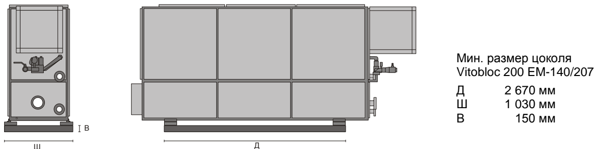
Рис. 7 БТЭС с цоколем
