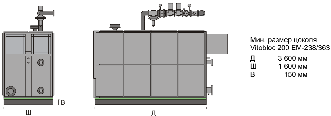
Рис. 7 БТЭС с цоколем
