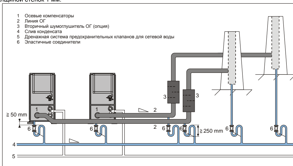
Рис. 12 Схема периферийной системы ОГ для двух модулей БТЭС с отводом конденсата и дренажной системой предохранительных клапанов (размеры в мм)
