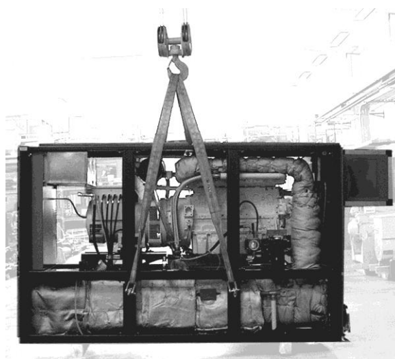
Рис. 4 Перемещение с помощью крана и канатов, требуется четыре дополнительные транспортировочные проушины
