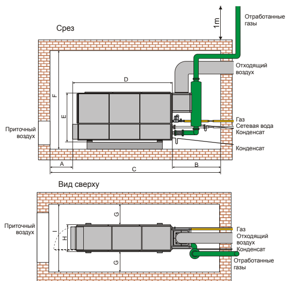
Рис. 6 Минимальные расстояния в рабочем помещении (размеры в мм)
