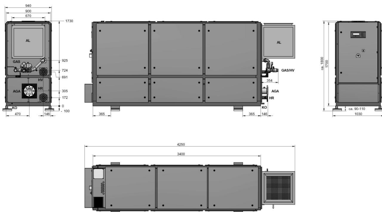
Рис. 1 Размеры и подключения модулей БТЭС Vitobloc 200 EM-140/207 (размеры в мм); уже смонтированный вентиляционный блок можно демонтировать для установки модуля
