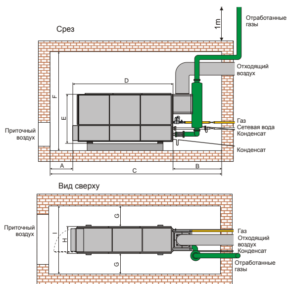
Рис. 9 Поддача приточного воздуха в рабочее помещение и отвод отходящего воздуха
