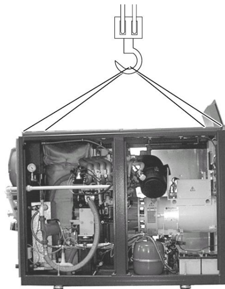
Рис. 3 Перемещение с помощью крана и канатов, требуется четыре дополнительные транспортировочные проушины
