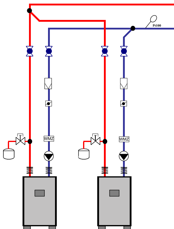
Рис. 10 Схема соединений гидравлического подключения
