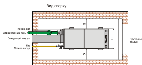
Рис. 8 Подача приточного воздуха в рабочее помещение и отвод отходящего воздуха
