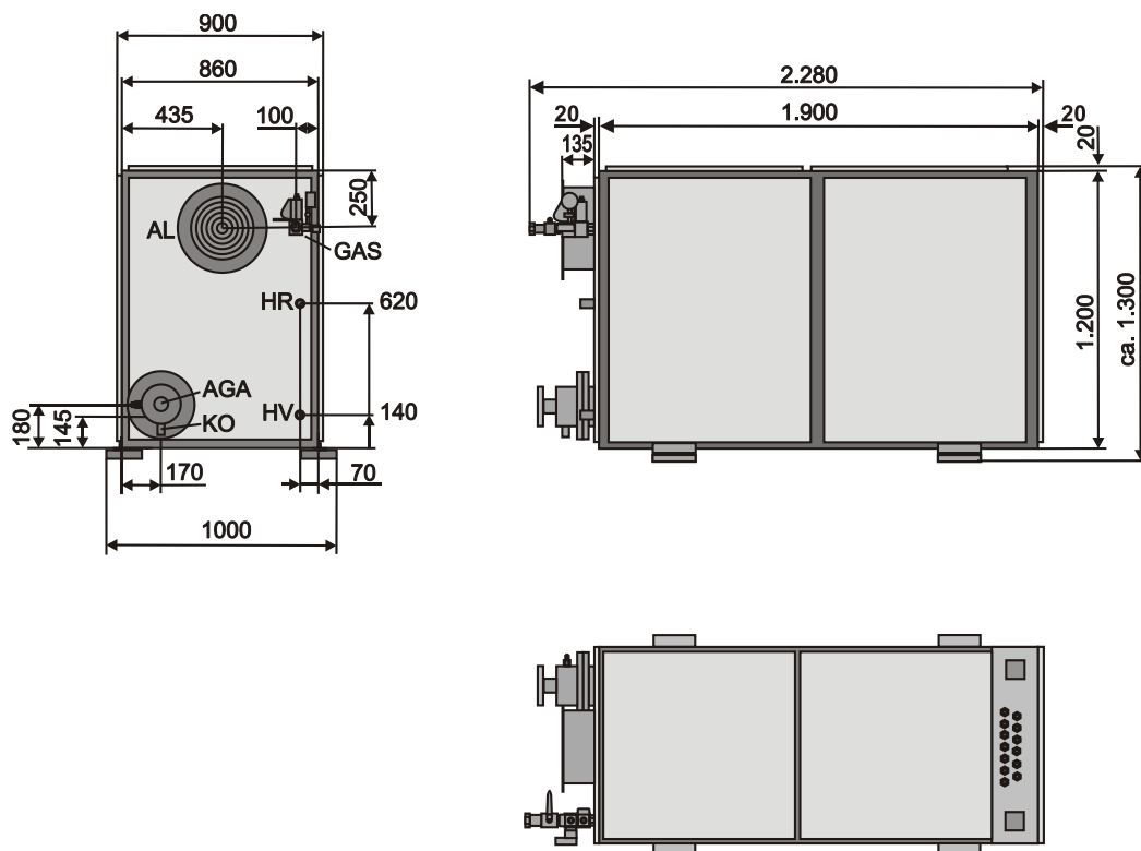
Рис. 1 Размеры и подключения модулей БТЭС Vitobloc 200 EM-18/36 (размеры в мм)
