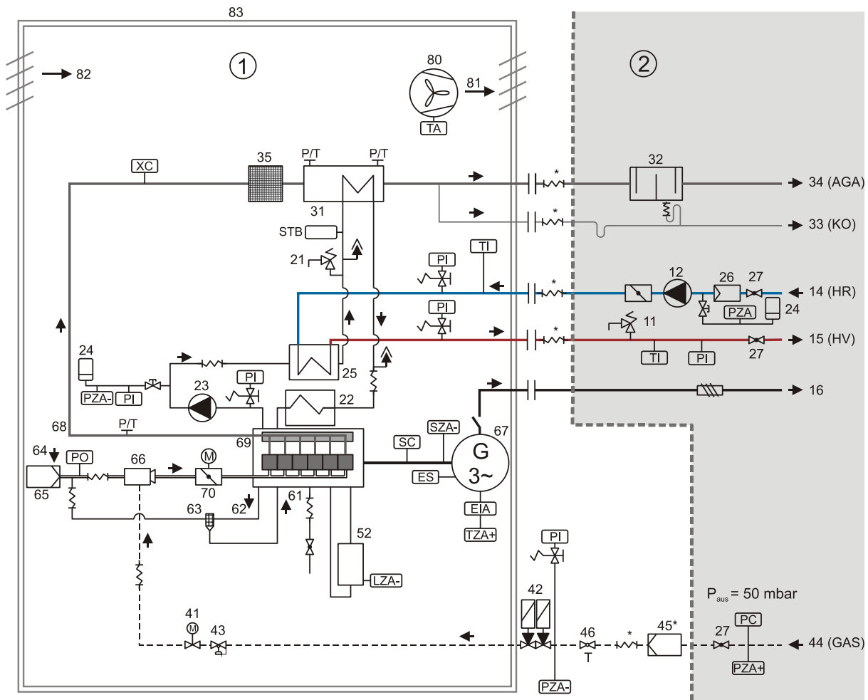
Рис. 7 Технологическая схема модуля БТЭС с возможностями периферийного подключения
