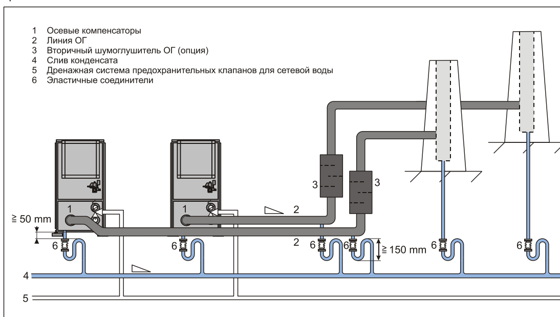
Рис. 11 Схема периферийной системы ОГ для двух модулей БТЭС с отводом конденсата и дренажной системой предохранительных клапанов (размеры в мм)
